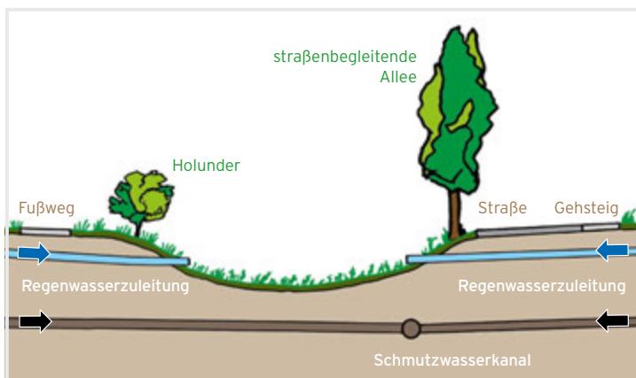
Abbildung 9 | Grünflächen entlang von Straßen, ausgebildet als Retentionsmulden, tragen zur Qualität einer Siedlung bei.
