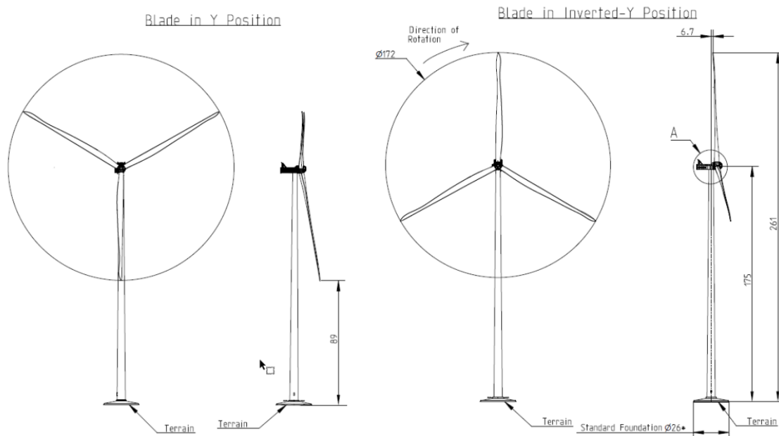
Abbildung 3: Vorder- und Seitenansicht Vestas V172 7,2 MW
